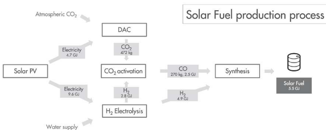
Figuur 4-3 Productieproces van synthetische brandstof op basis van zonne-energie (Power-to-Liquid of PtL). DAC=Direct Air Capture. Overgenomen uit:(Kraan, Kramer, Haigh, & Laurens, 2019).
